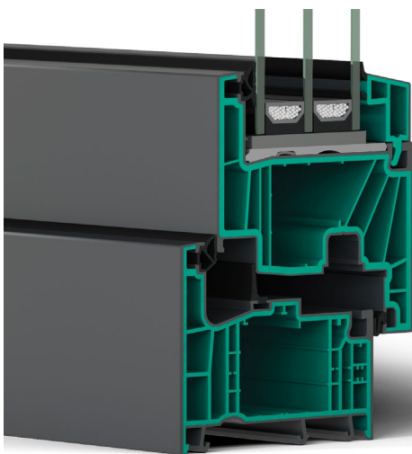
Rezyklate im ARTEVO Profilkern sowie in den Glasleisten
